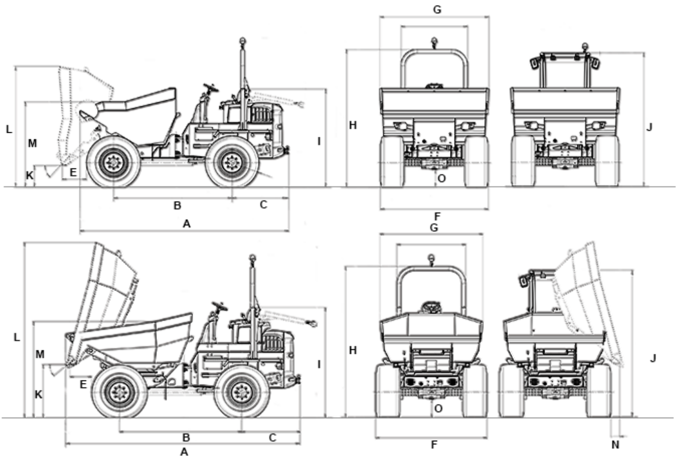
DW60 Frontkipplader DW60 Drehkipplader DW60 Power Drehkipplader
